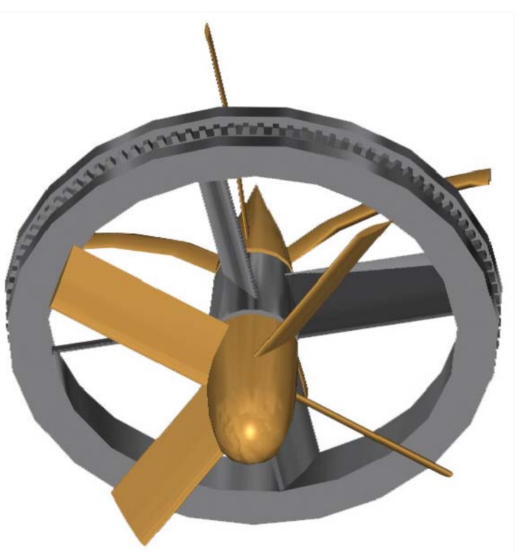
Estator, rotor, buje y soporte posterior, aislados
